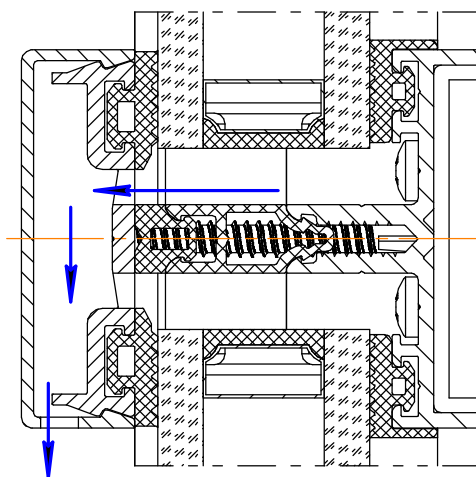
Б-Б Водоотвод
