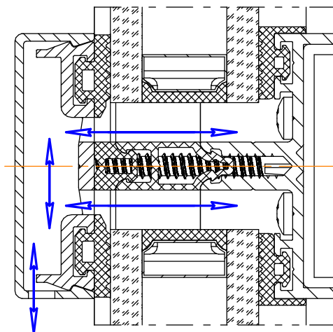
Б-Б Вентиляция
