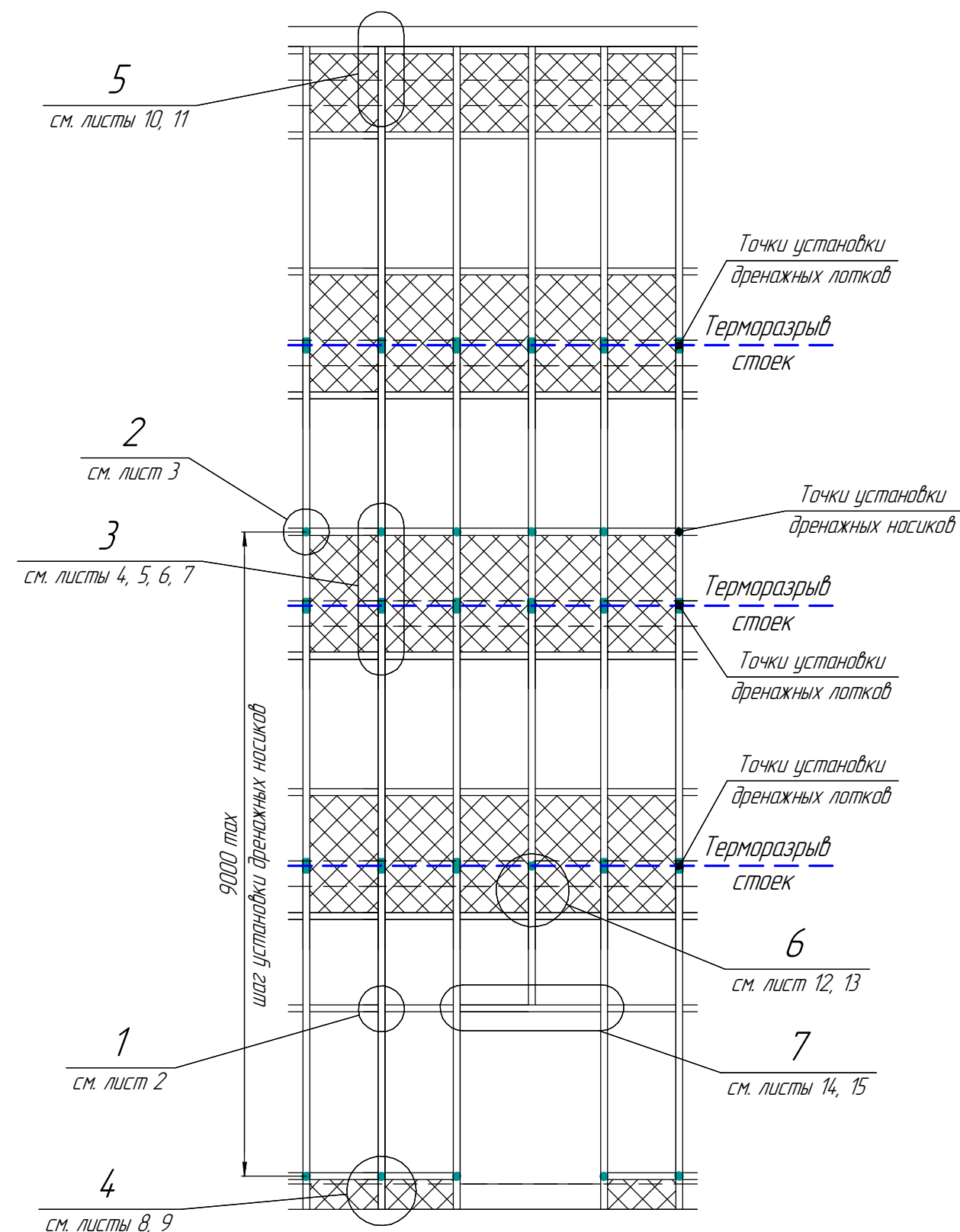
Схема расположения основных узлов плоского участка фасада FA50-K50
